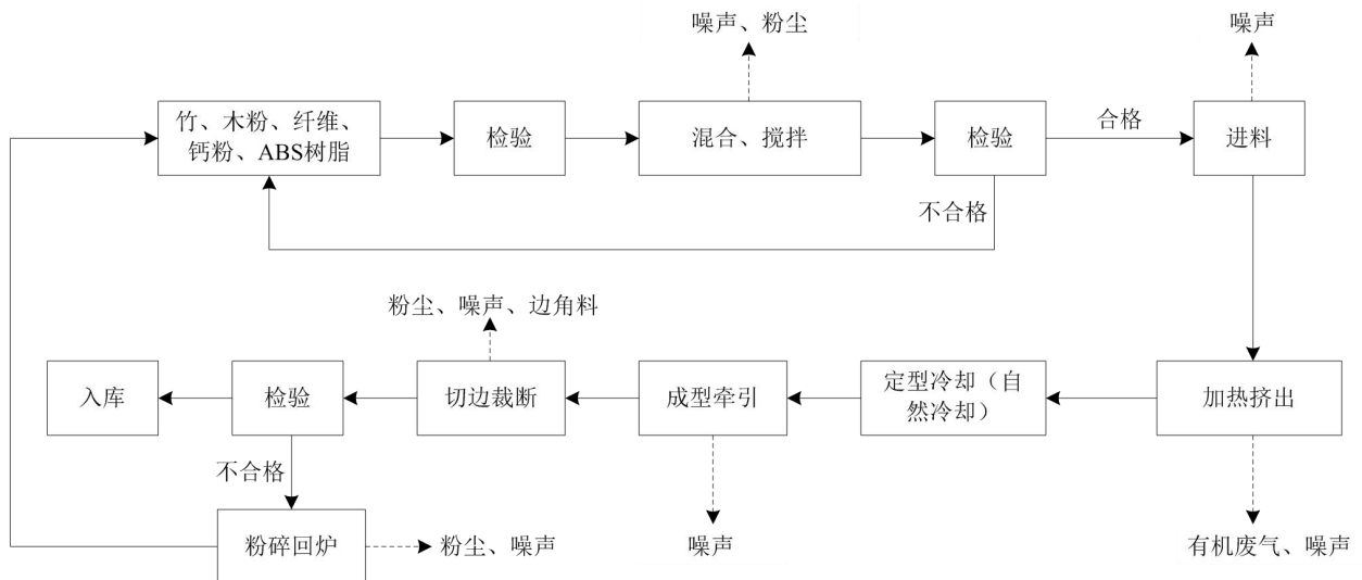
图 4.3-2 竹木纤维护墙板生产工艺图
