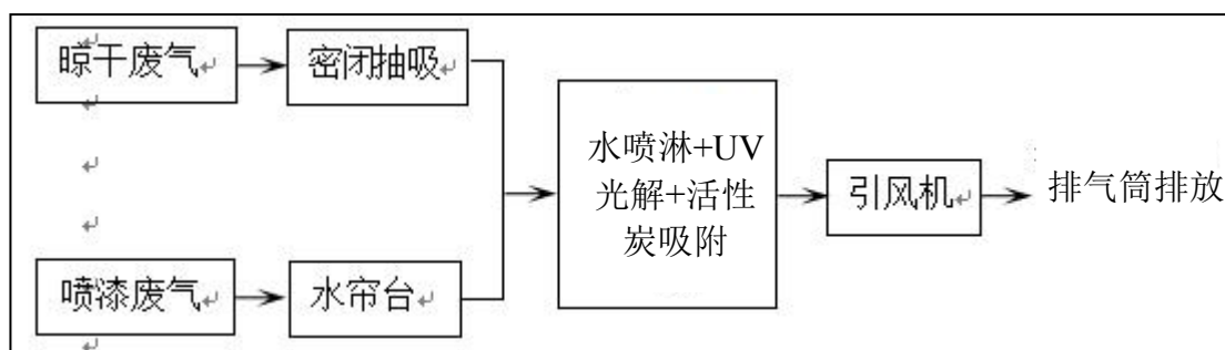
图 8.2-2 涂装废气处理工艺图
