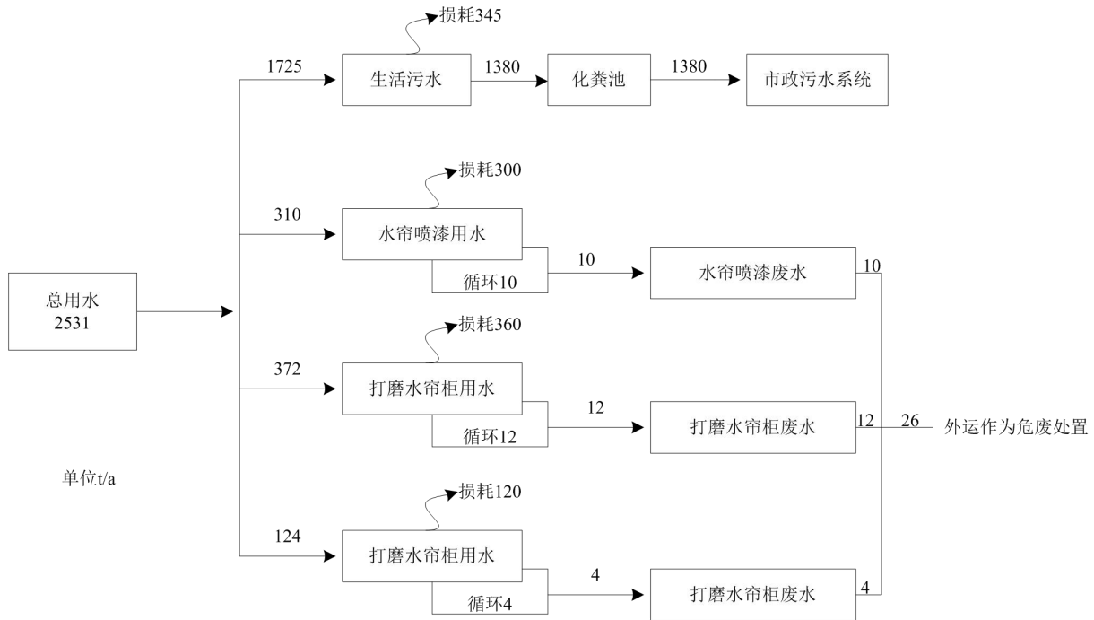
图 4.5-2 项目水平衡图（单位： \text{m}^3/\text{a} ）
