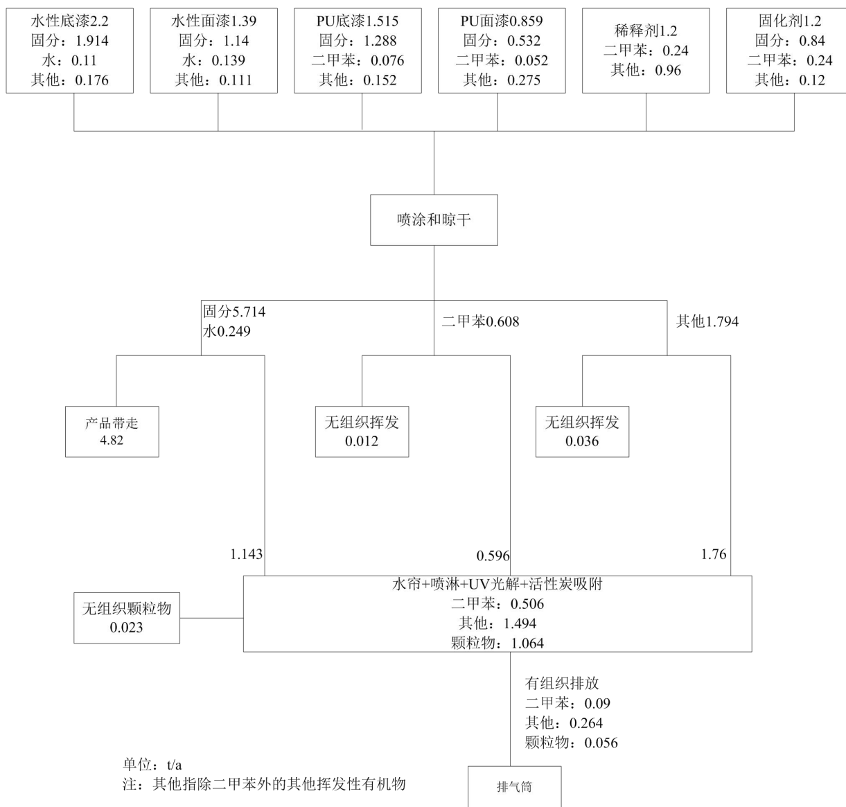
图 4.5-1 油漆物料平衡图
