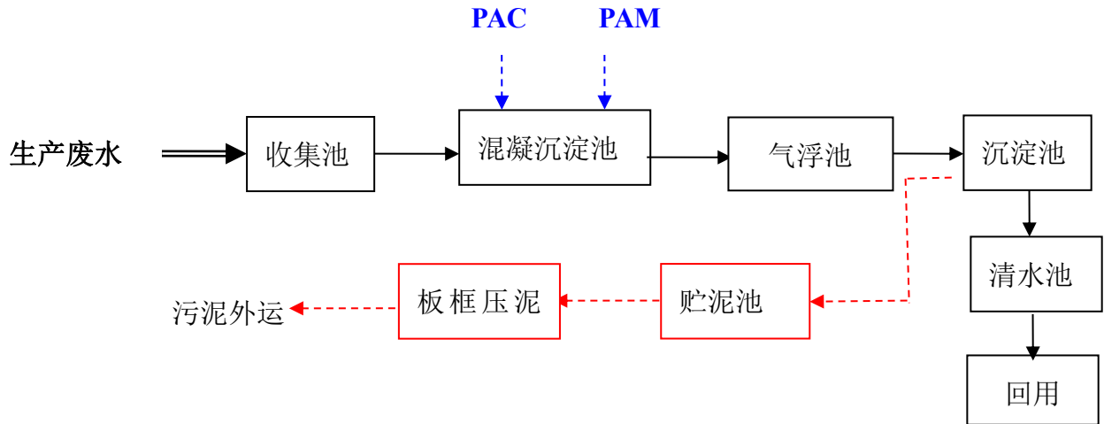
图 8.2-1 生产废水处理工艺流程图
