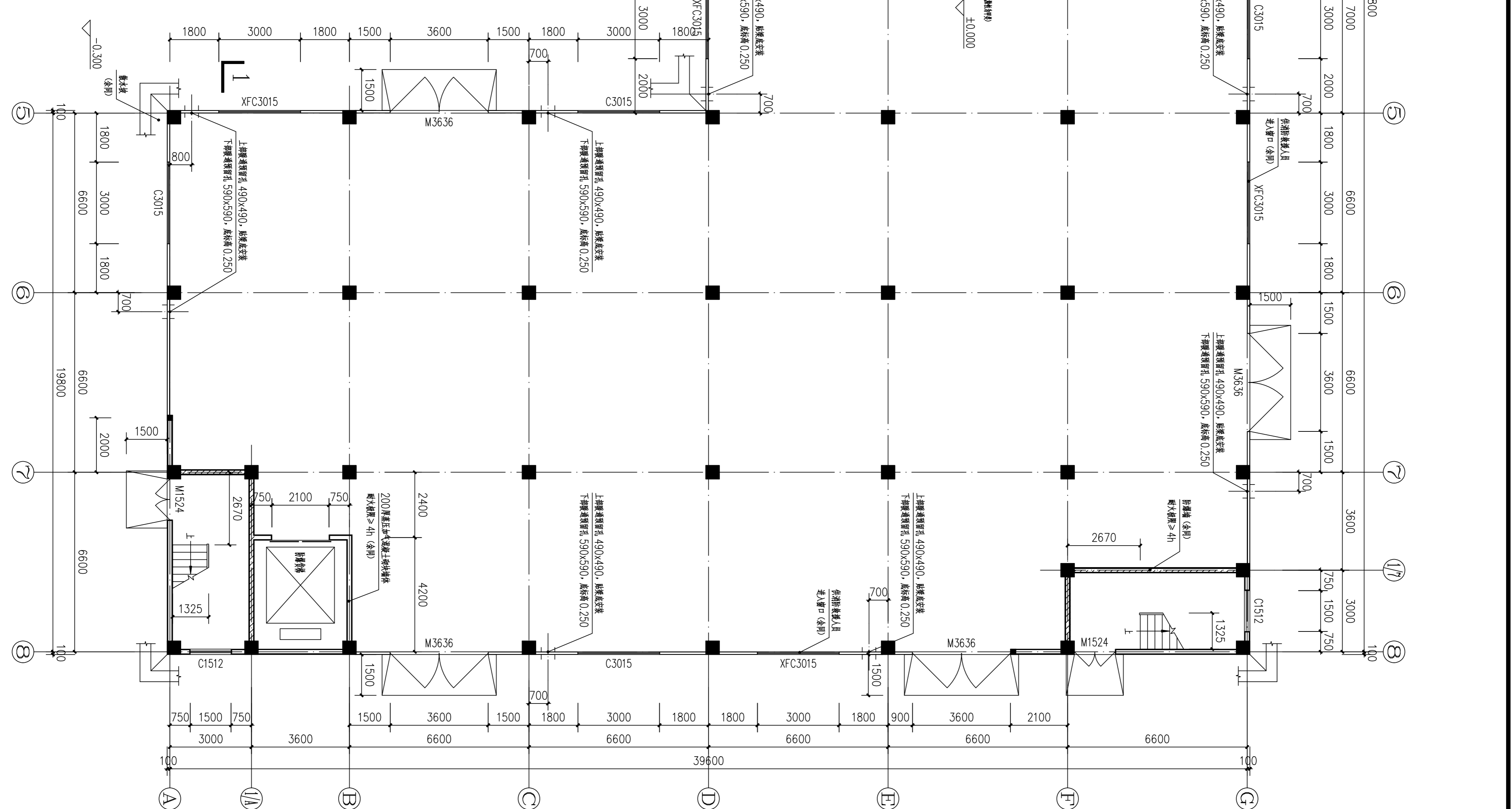
±0.000标高平面图 1:100
